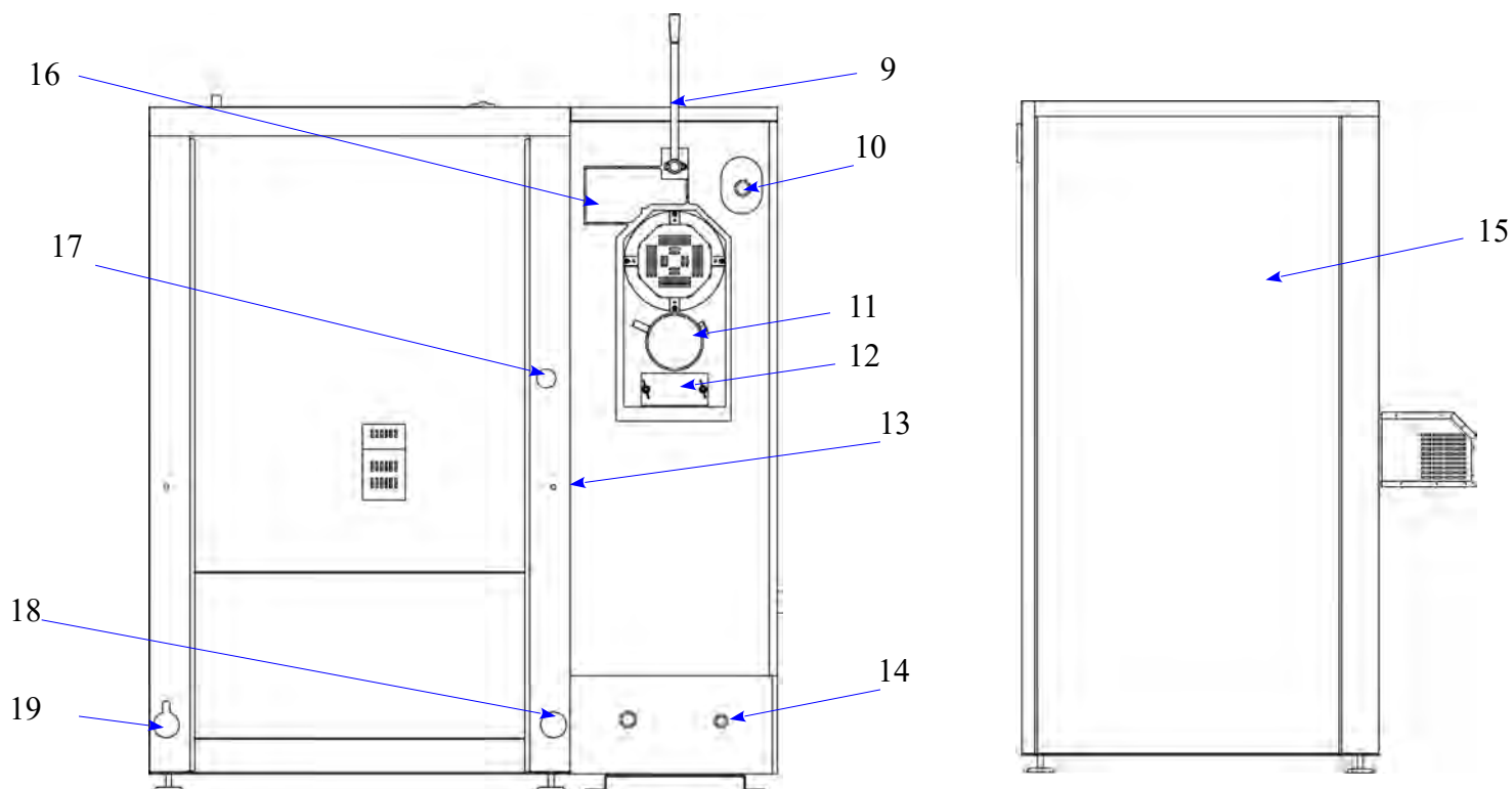
Zeichnung nr 5. Schematische Übersicht der Kessel Bautypen Smart Fire SF 11, SF15, SF15/3bar, SF22, SF22/3bar, SF31 und SF41:
