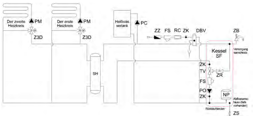
Zeichnung nr 38. Geschlossener Kreislauf + WW > 220L + 2 Kreislauf am 3D-Ventil
