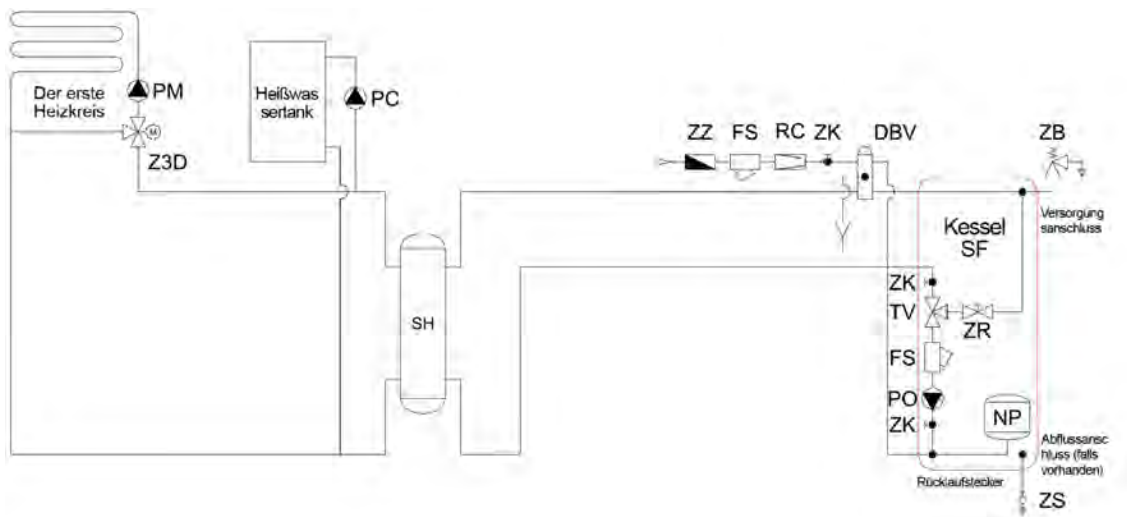
Zeichnung nr 33. Geschlossener Kreislauf + WW > 220L + 1 Kreislauf am 3D-Ventil
