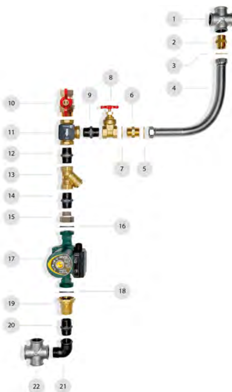
Zeichnung nr 41. Hydraulikset der Kessel Smart Fire Kessel SF15/3bar, SF22, SF22/3bar, SF31 und SF41:
