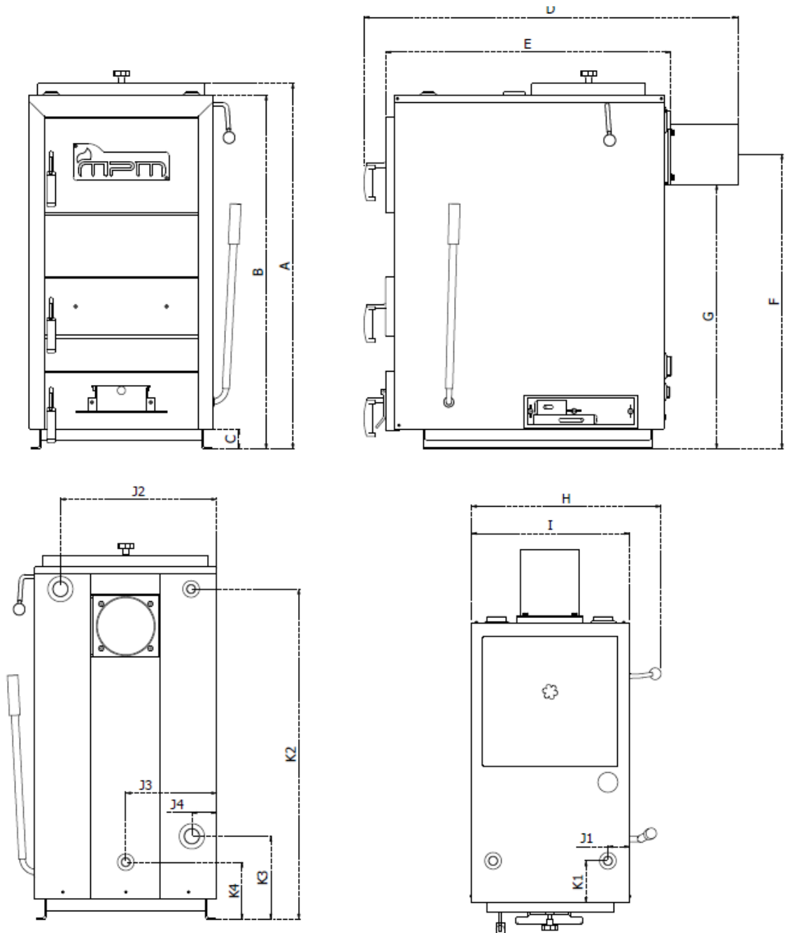
Abbildung 2: Grundlegende Abmessungen des MPM Wood Plus Holzkessels
