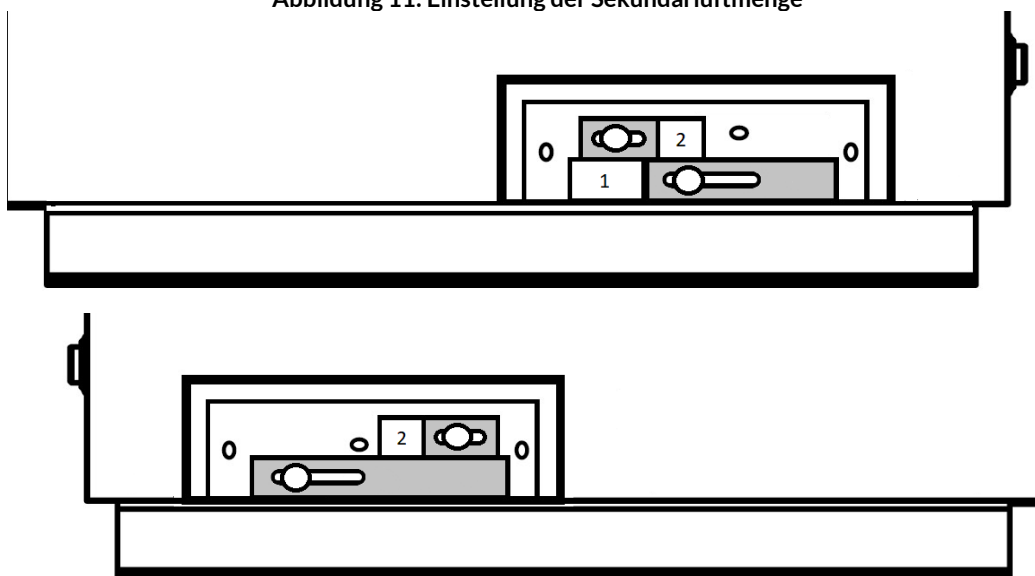
Abbildung 11: Einstellung der Sekundärluftmenge
