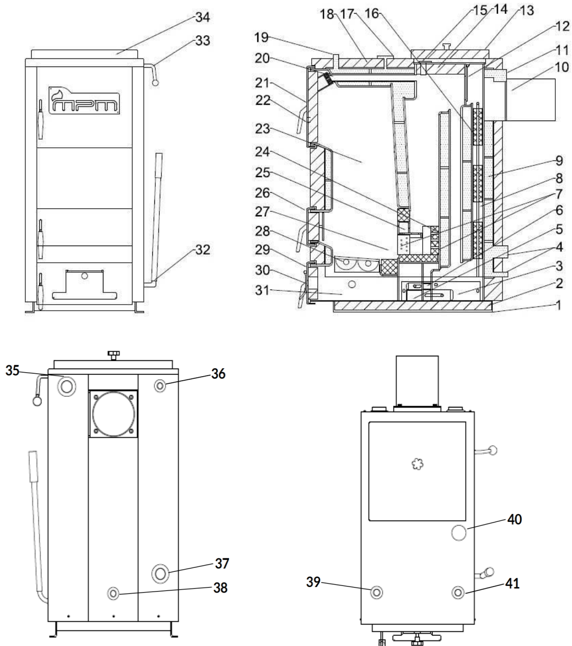
Abbildung 1: Schematische Darstellung eines Seitenladerkessels
